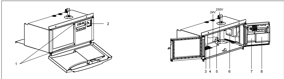
afb. 15 Gesloten en geopende instrumentenkast pdf
