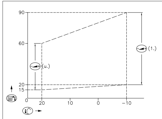
afb. 20 Interne stooklijn 00.W4H.79.00017
