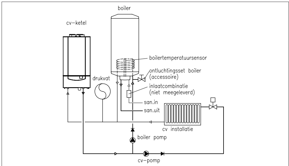
afb. 11 Aansluiting boiler m.b.v. boilerpomp.
