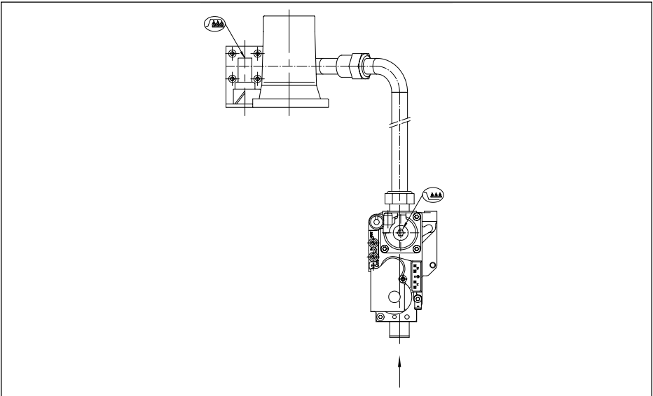
Afb. 27 Instelpunten 00.W3H.79.00050
