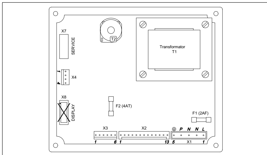
Afb. 18 Beveiligingsautomaat Gasmodul met reservezekeringen
