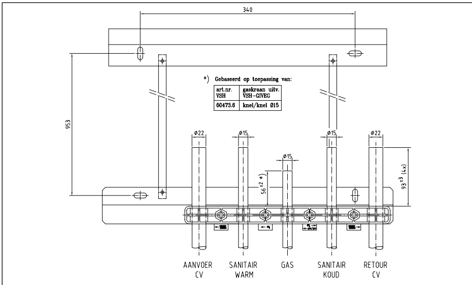
Afb. 08 Montagebeugel (optie)
