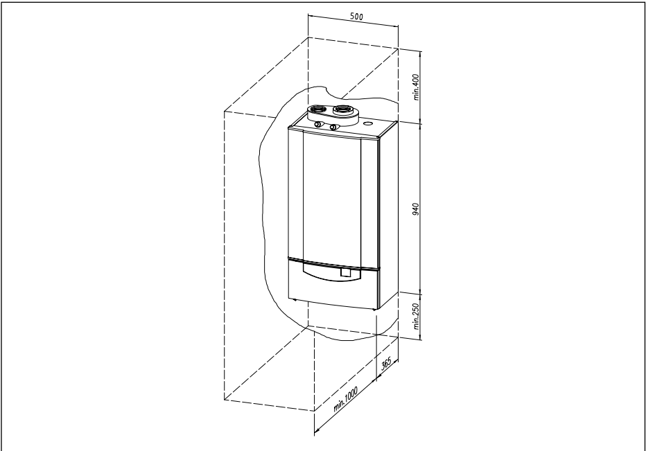
Afb. 07 Opstellingsruimte Remeha Quinta 00.W3H.79.00040
