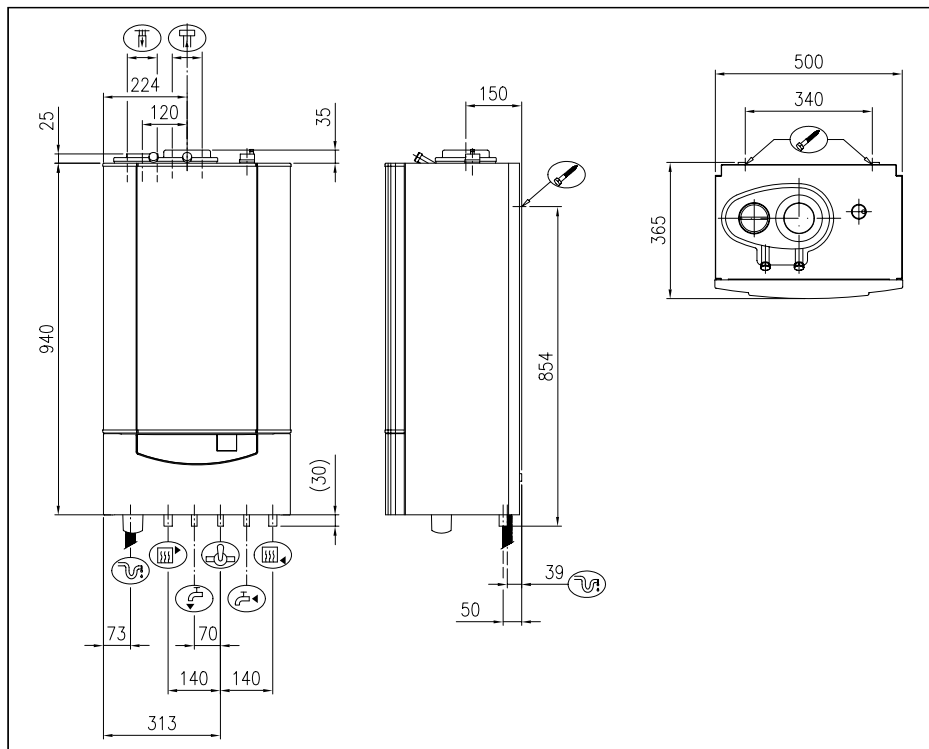
Afb. 03 Afmetingen Remeha Quinta 28c en Quinta 35c
