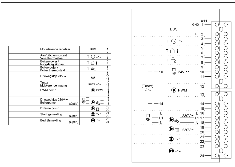
Afb. 19 Klemmenstrook 00.W3H.79.00059
