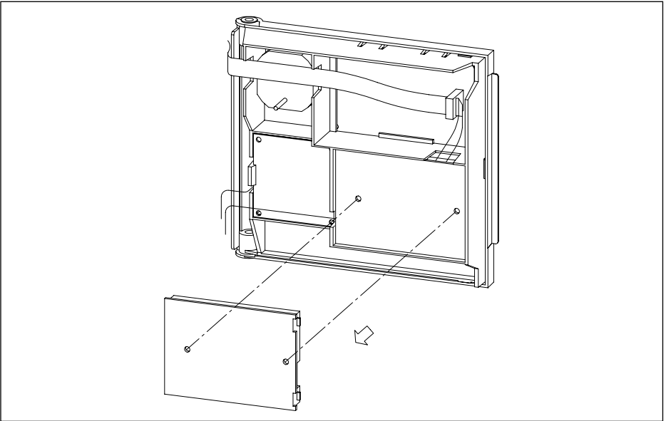
Afb. 21 Interface inbouw 05.W4H.79.00008
