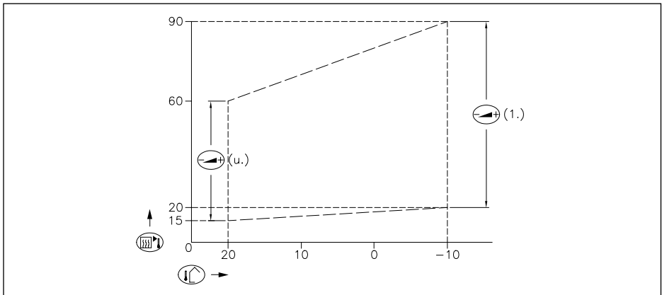
Afb. 24 Interne stooklijn 00.W4H.79.00017
