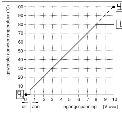
Afb. 22 Relatie tussen ingangsspanning en ketelaanvoertemperatuur
