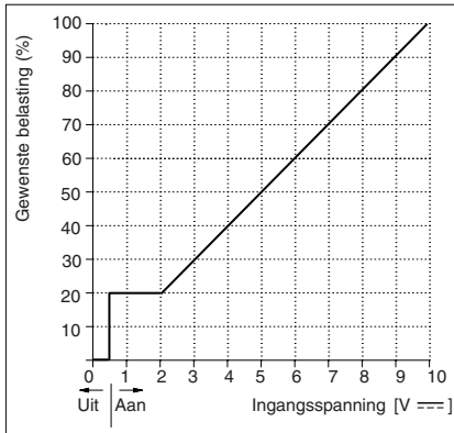
Afb. 23 Relatie tussen ingangsspanning en nominale belasting
