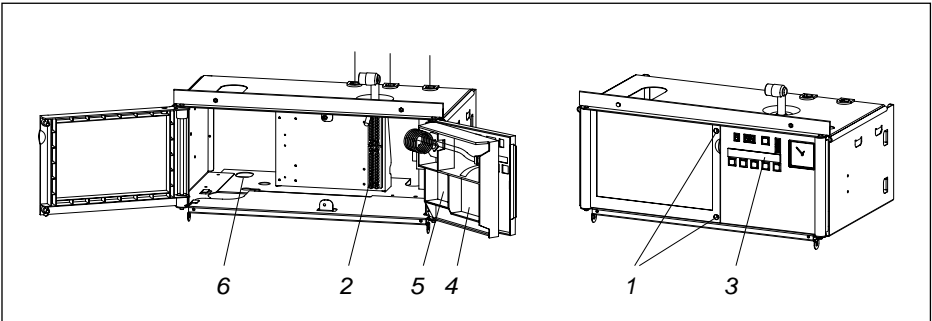
Afb. 20 Gesloten en geopende instrumentenkast 00.W3H.79.00054
