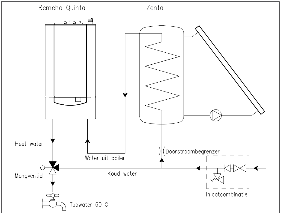
Afb. 17 Principeschema Remeha Quinta 28c of Quinta 35c met Remeha Zenta zonneboiler
