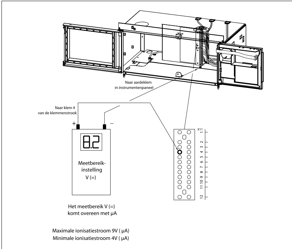
Afb. 29 Ionisatiemeting 00.W3H.79.00051
