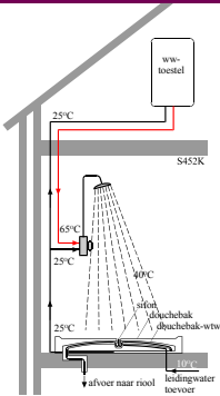
Werking van douche-waterwarmtewisselaar.
