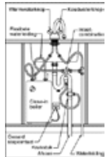
Werking van close-in boiler met cold fill en met hot fill.
